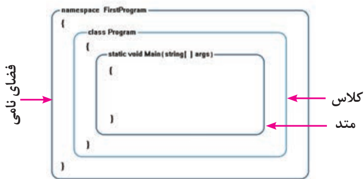
شکل ۱۰- الگوی یک برنامه ساده سی شارپ
